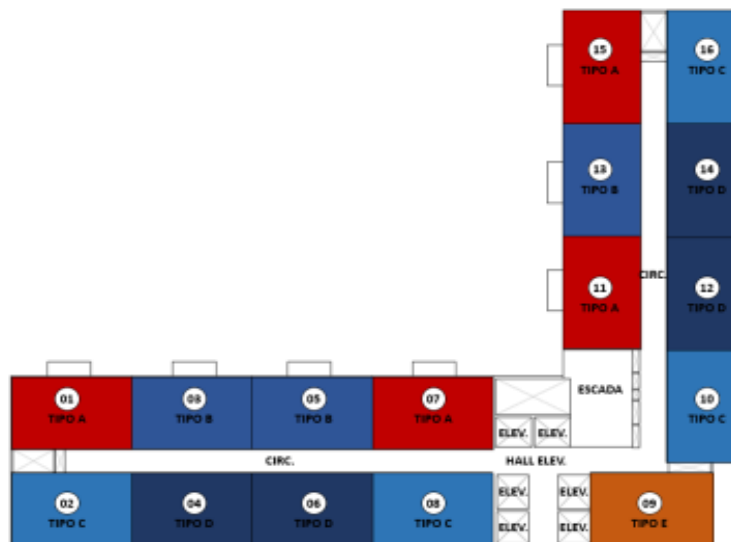
PLANTA 3º AO 18º PAVIMENTO
